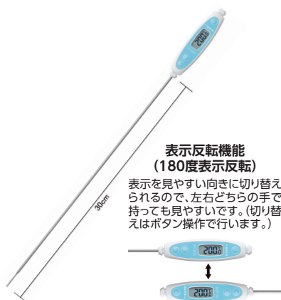
C512-04 表示反転機能付防水型デジタル温度計 Drip Proof Digital Thermometers
