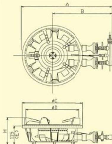
■ MG-260B、270B、280B、290B 尺寸图
