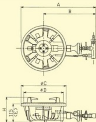
■ MG-240C、250B 尺寸图
